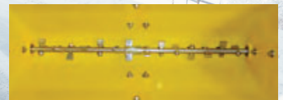
robuste Rührwelle, Achse mittig geteilt, einstellbare Rührflügel
