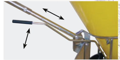
Schalthebel und verstellbare Schubstange
