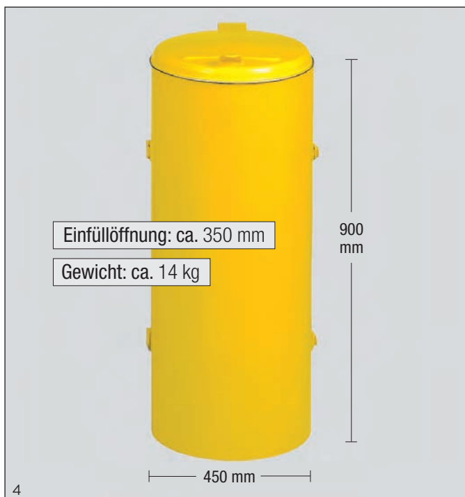
Abb.: Kompakt-Junior mit Einflügeltür, gelb beschichtet, Art.-Nr. 1017
