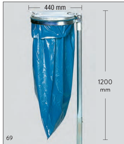
Abb.: Modell „Stationär mit Verschraubung, verzinkt“ mit ME-Deckel, Art.-Nr. 10311
